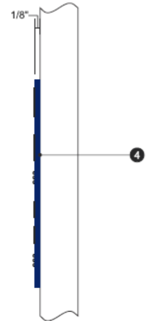
Side View Scale: 1/2 of Actual Size
